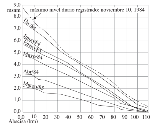
Figura 16. Niveles promedio mensuales
