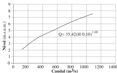
Fig 18. Curva de calibración del Canal del Dique, km 6,5–7,0
