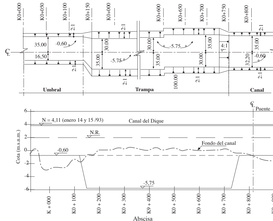
Figura 7. Planta (arriba) y perfil de la trampa de Calamar
