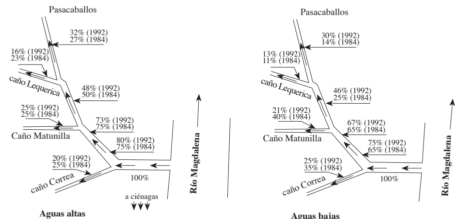
Figura 19. Distribución de caudales líquidos en bifurcaciones. 1984–1992
