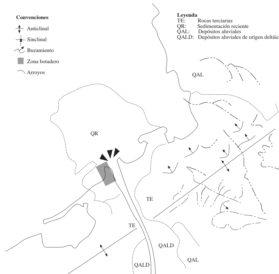
Figura 14. Geomorfología de la zona de Pasacaballos, 1991
